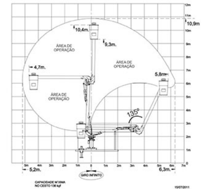
Diagrama Operacional de Cargas e Alcances
