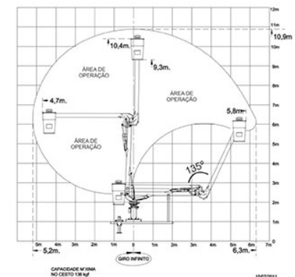
Diagrama Operacional de Cargas e Alcances
